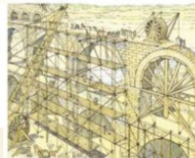
3 Bouwwerf van een aquaduct. Constructies zoals aquaducten worden gebouwd door grote blokken natuursteen op elkaar te zetten, zonder mortel! De blokken worden vastgemaakt met ijzeren krammen.
